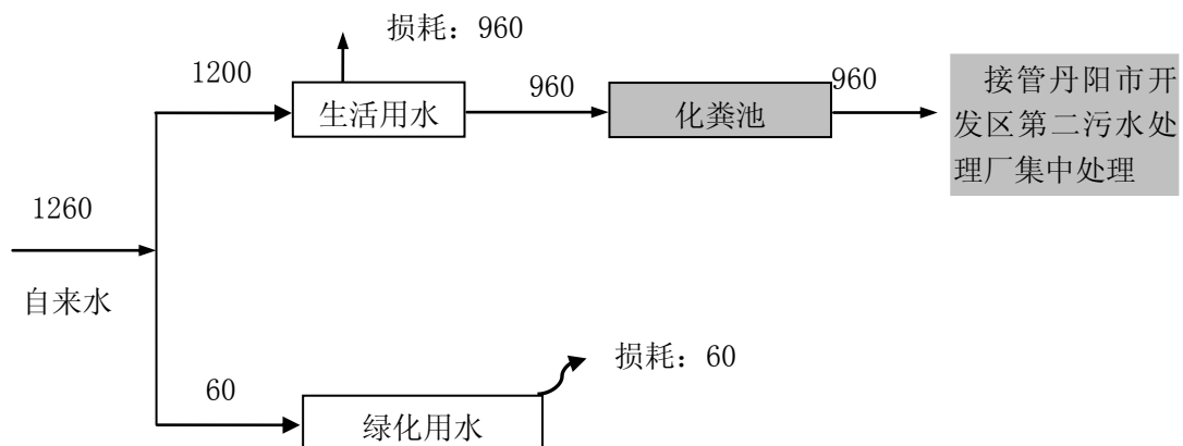
图 2 本项目水量平衡图（单位：m 3 /a）
