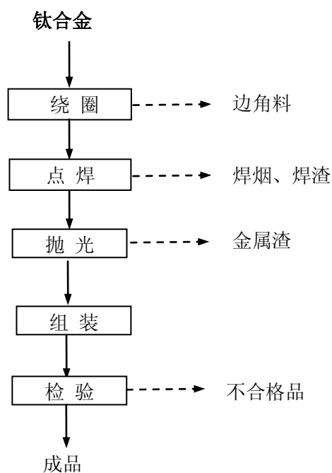
图1 生产工艺流程及产污环节图
