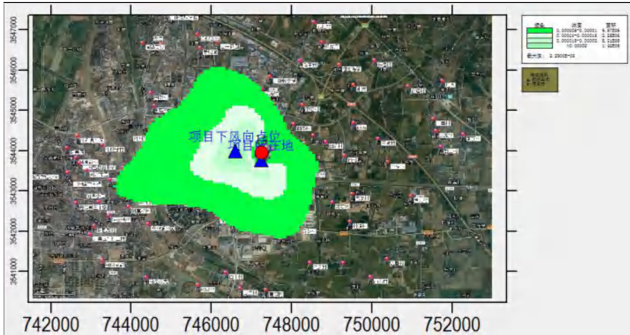
图6.1.3-4PM10贡献质量浓度预测（年均值）
