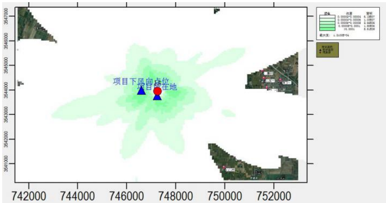
图6.1.3-3PM10贡献质量浓度预测（日均值）
