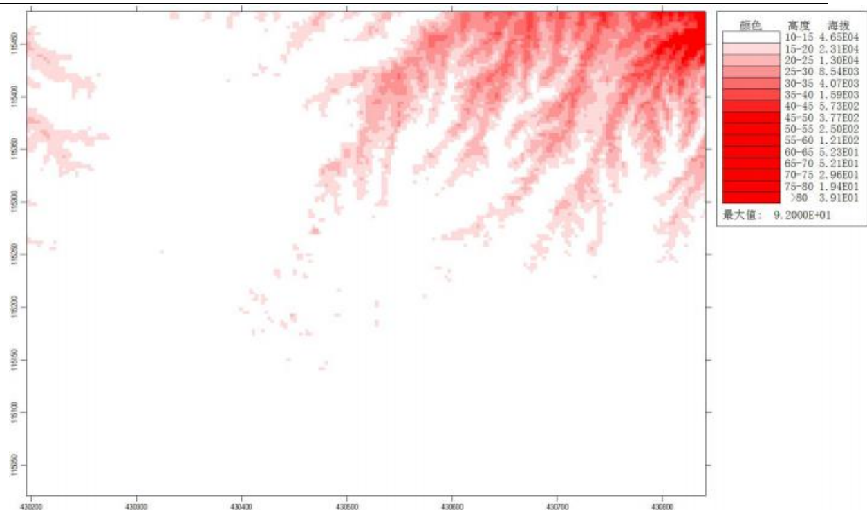
图6.1.3-1区域等高线示意图
