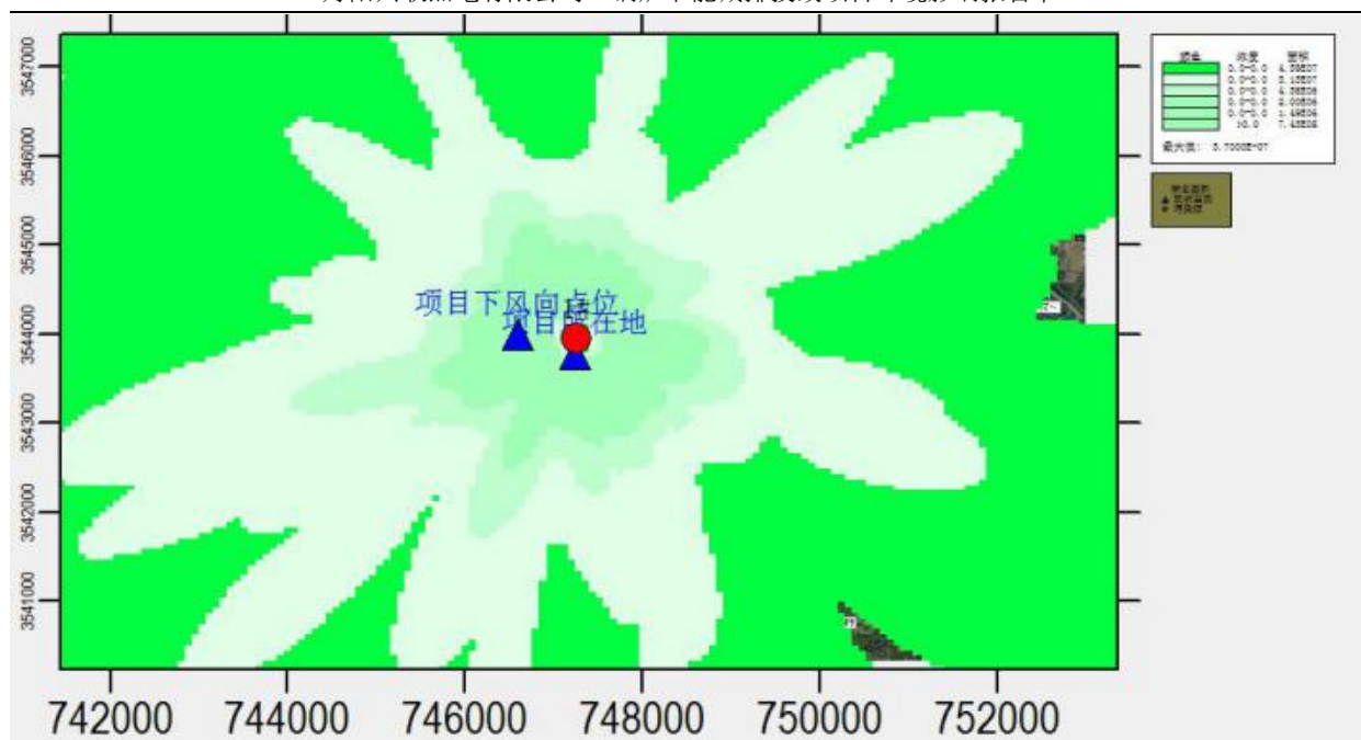
图6.1.3-6汞贡献质量浓度预测（日均值）
