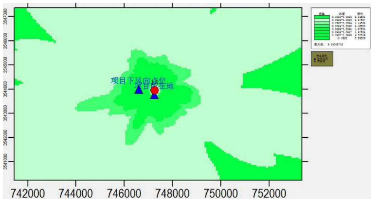
图6.1.3-9二氧化氮贡献质量浓度预测（日均值）
