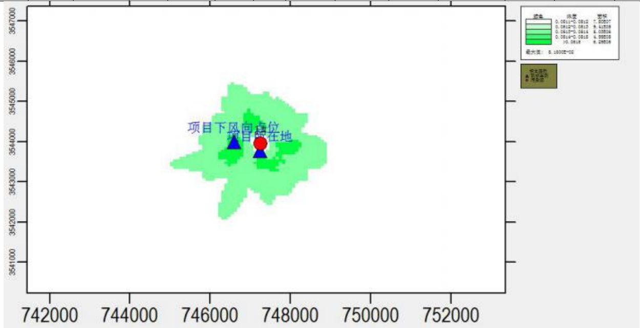
图6.1.3-7二氧化硫贡献质量浓度预测（日均值）
