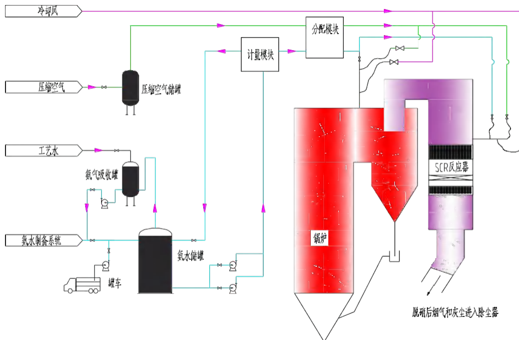
图7.1-3 SNCR/SCR联合工艺脱硝流程图
