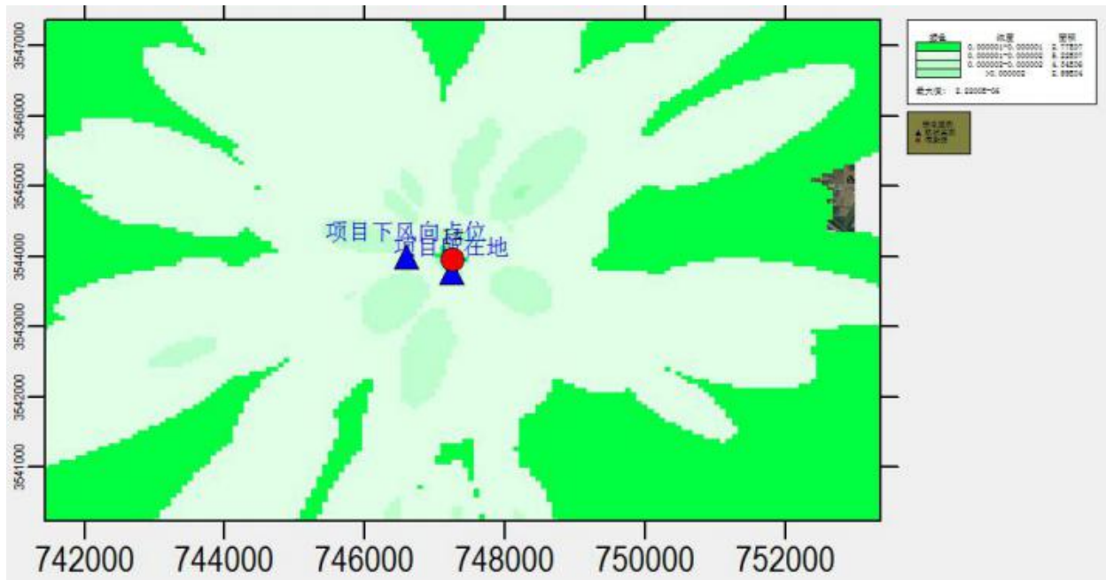
图6.1.3-5汞贡献质量浓度预测（小时值）
