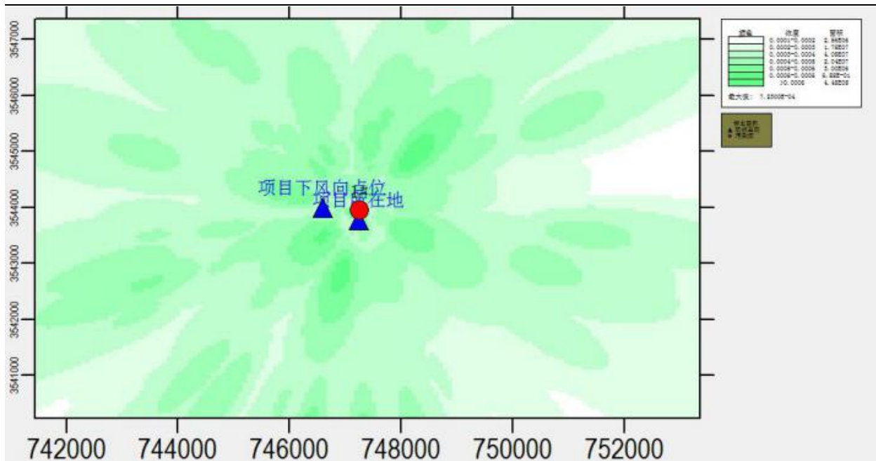
图6.1.3-2PM10贡献质量浓度预测（小时值）
