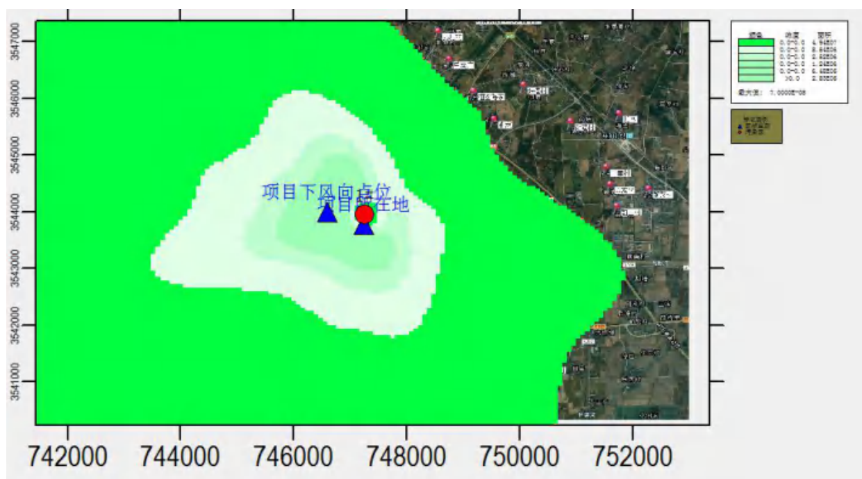
图6.1.3-7汞贡献质量浓度预测（年均值）
