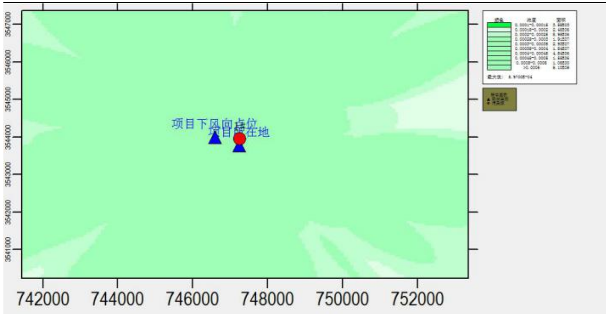
图6.1.3-4氨贡献质量浓度预测（小时值）
